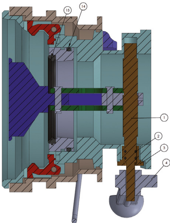
SECCIÓN AG-AG ESCALA 1 : 2
